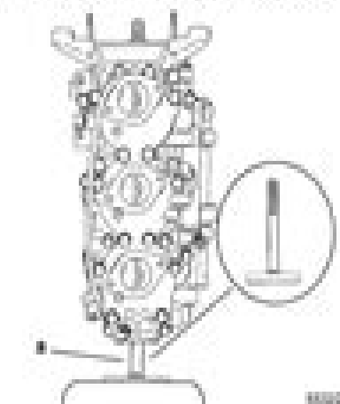
a - Powerhead Stand (31-62700-1-1) (40700) shown Powerhead Stand (31-20627-1-1) (30400)
