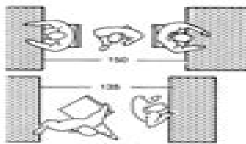
3 Mindest-Spielraum im Lesebereich → 4
