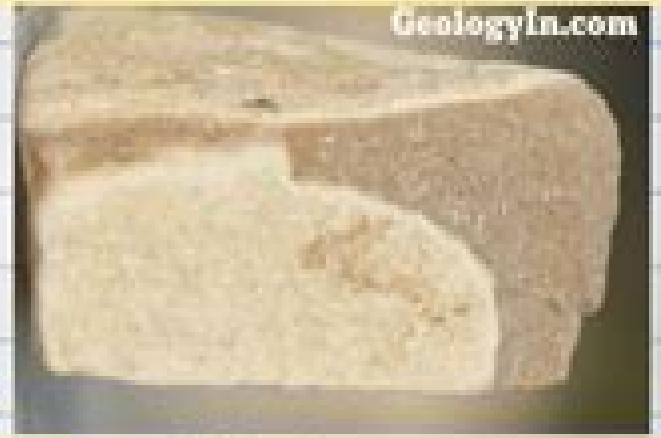
Mudstone
