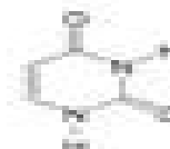
Uracil
