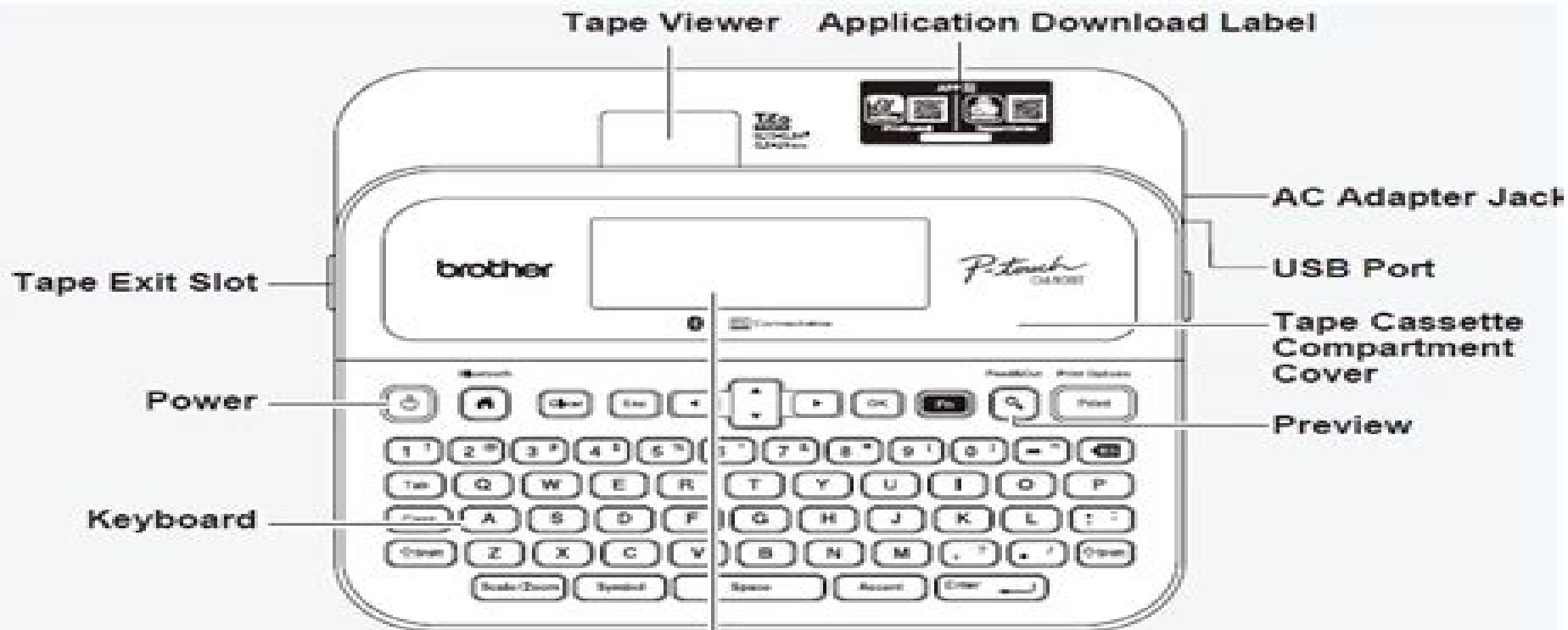
LCD
